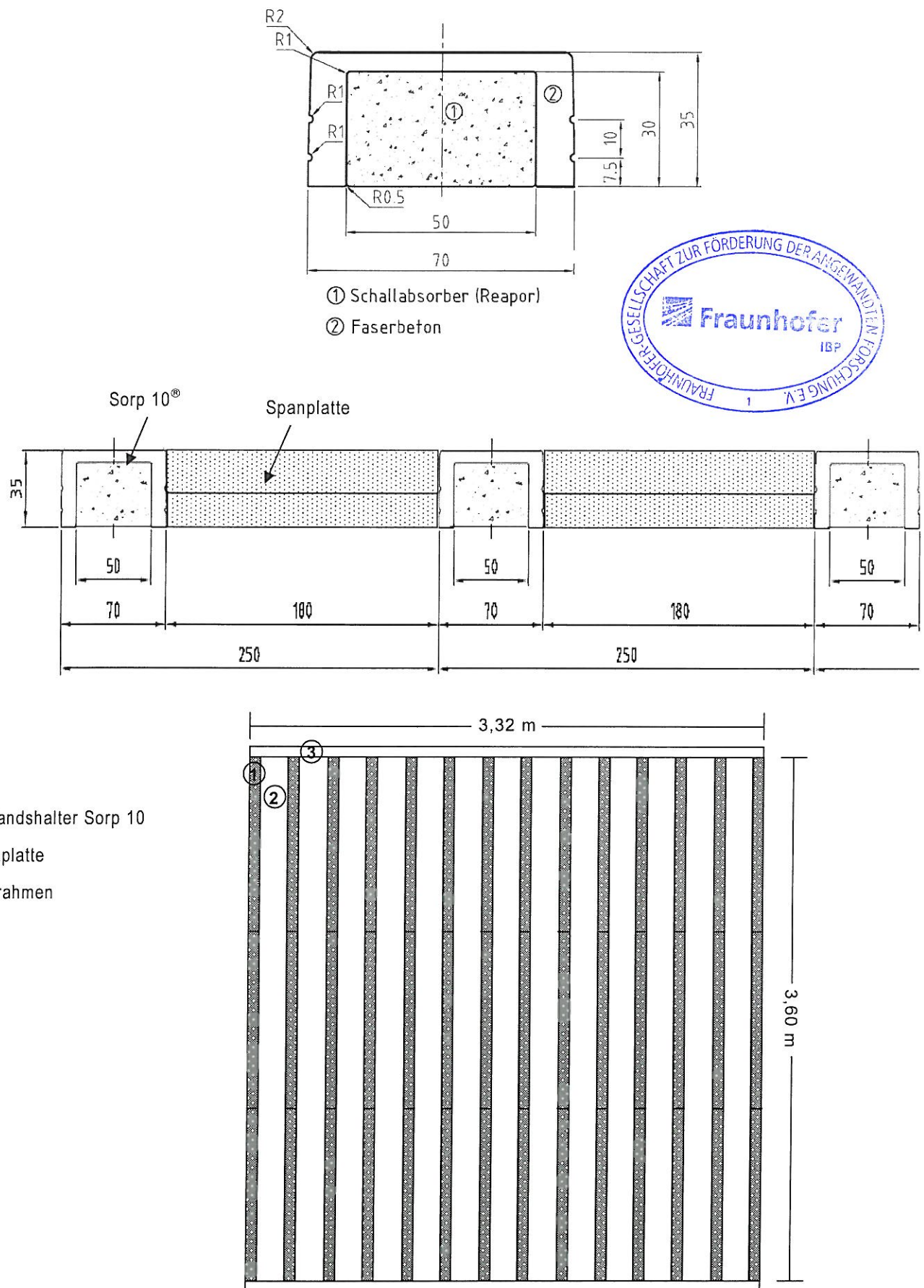
Bild 2 Detailzeichnungen (Schnitt durch einen Abstandshalter Schnitt durch den Prüfaufbau) sowie Ansicht des Prüfaufbaus im Hallraum; (Prüfobjekt S 10362-01; Maße in Millimeter (mm)).
